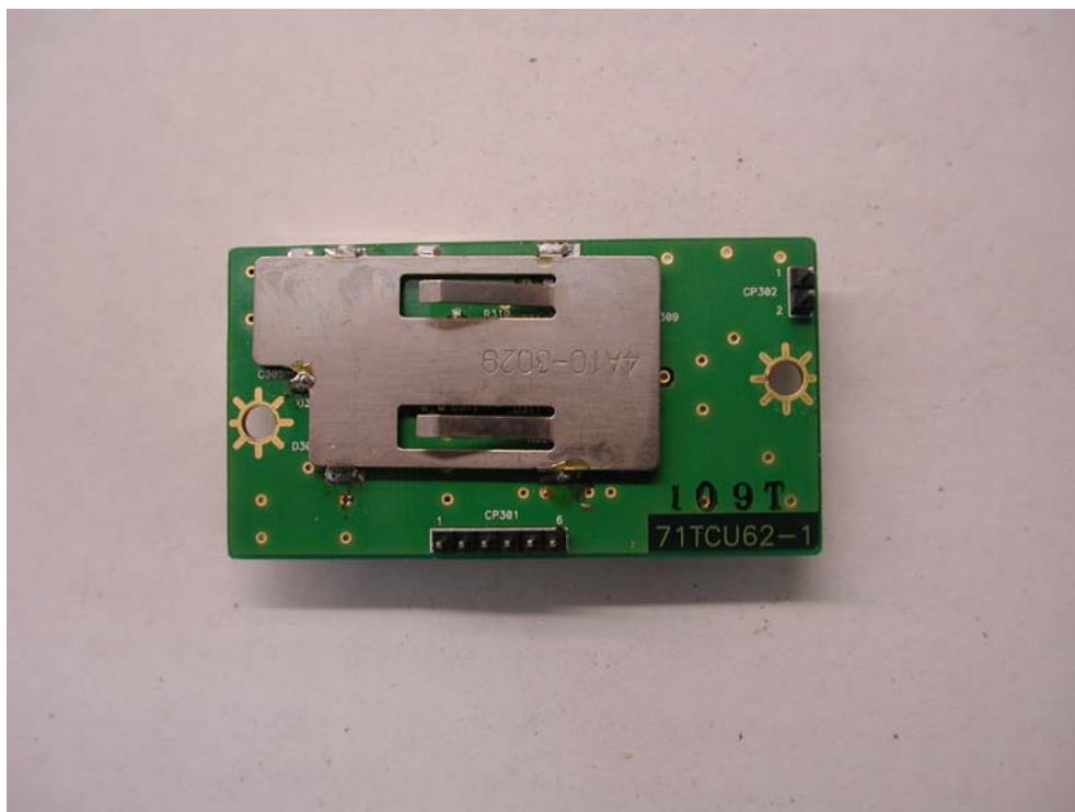
RX VCO BOTTOM
