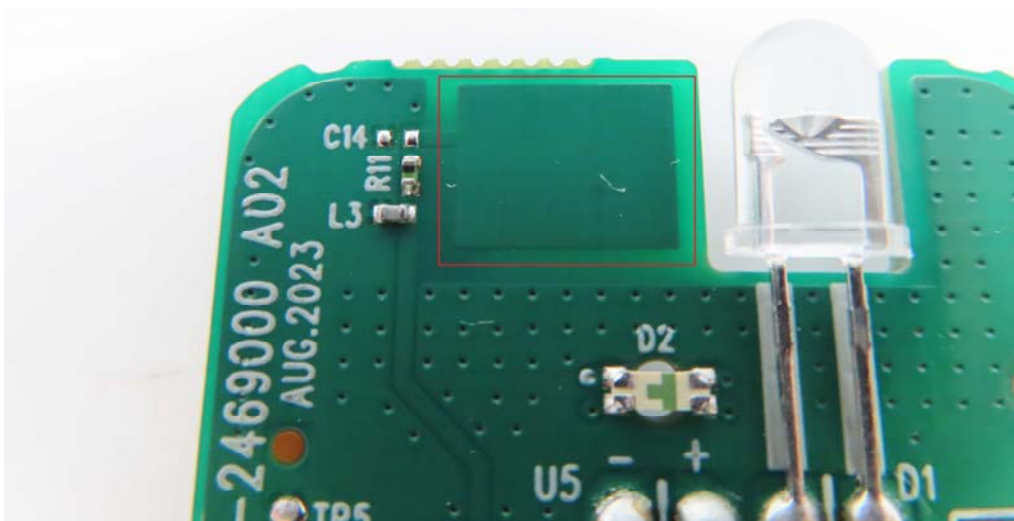
BLE&Zigbee Module
