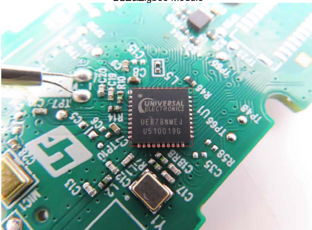
BLE&Zigbee Module
