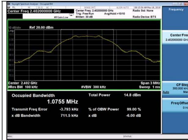
6dB BW –Bluetooth LE 2402MHz
