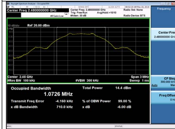
6dB BW –Bluetooth LE 2480MHz
