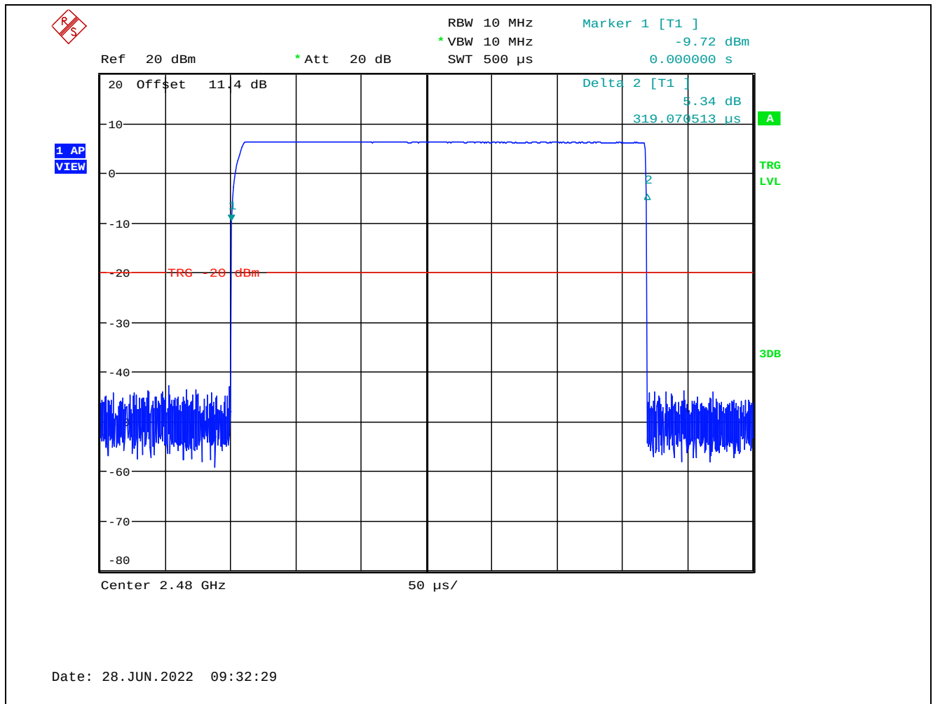
Plot 5.3.3.1.3. Duty Cycle (Pulse)
