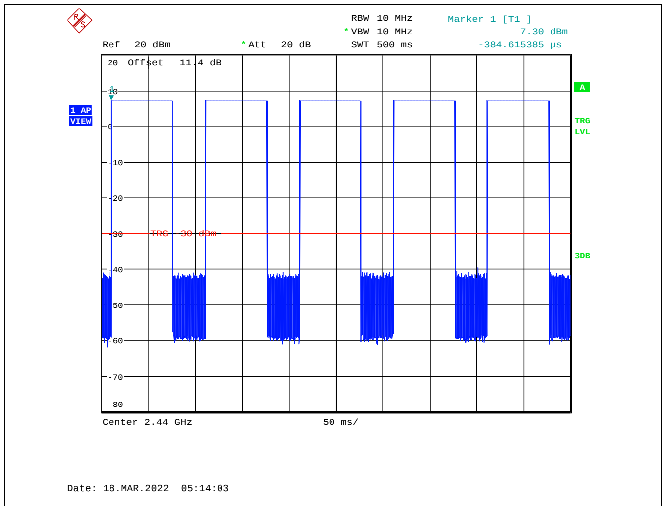
Plot 5.7.4.1.1. Duty Cycle (Pulse Train)
