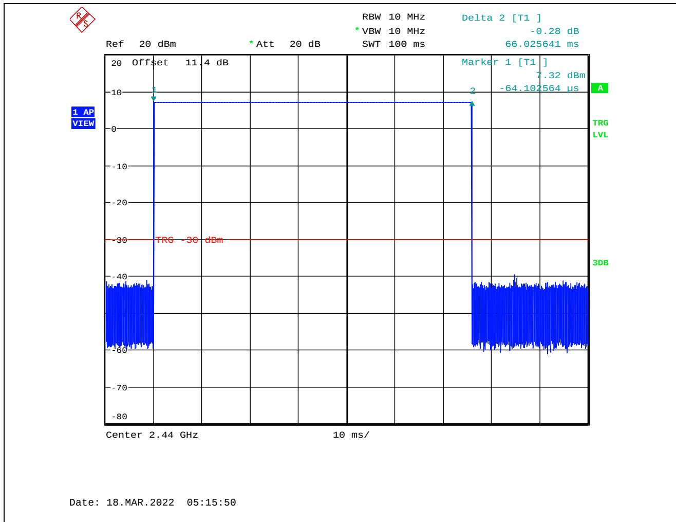
Plot 5.7.4.1.3. Duty Cycle (Pulse)
