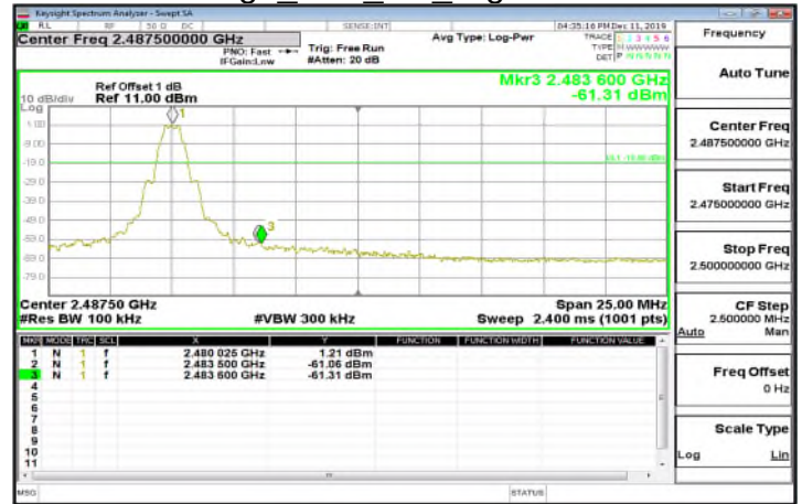
Band Edge BLE 1M HighCH39-2480
