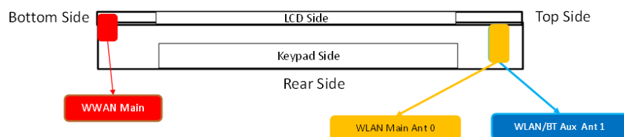
<EUT Right Side>
