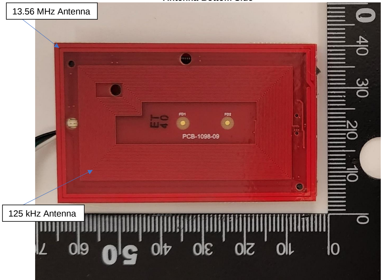
Antenna-Bottom Side
