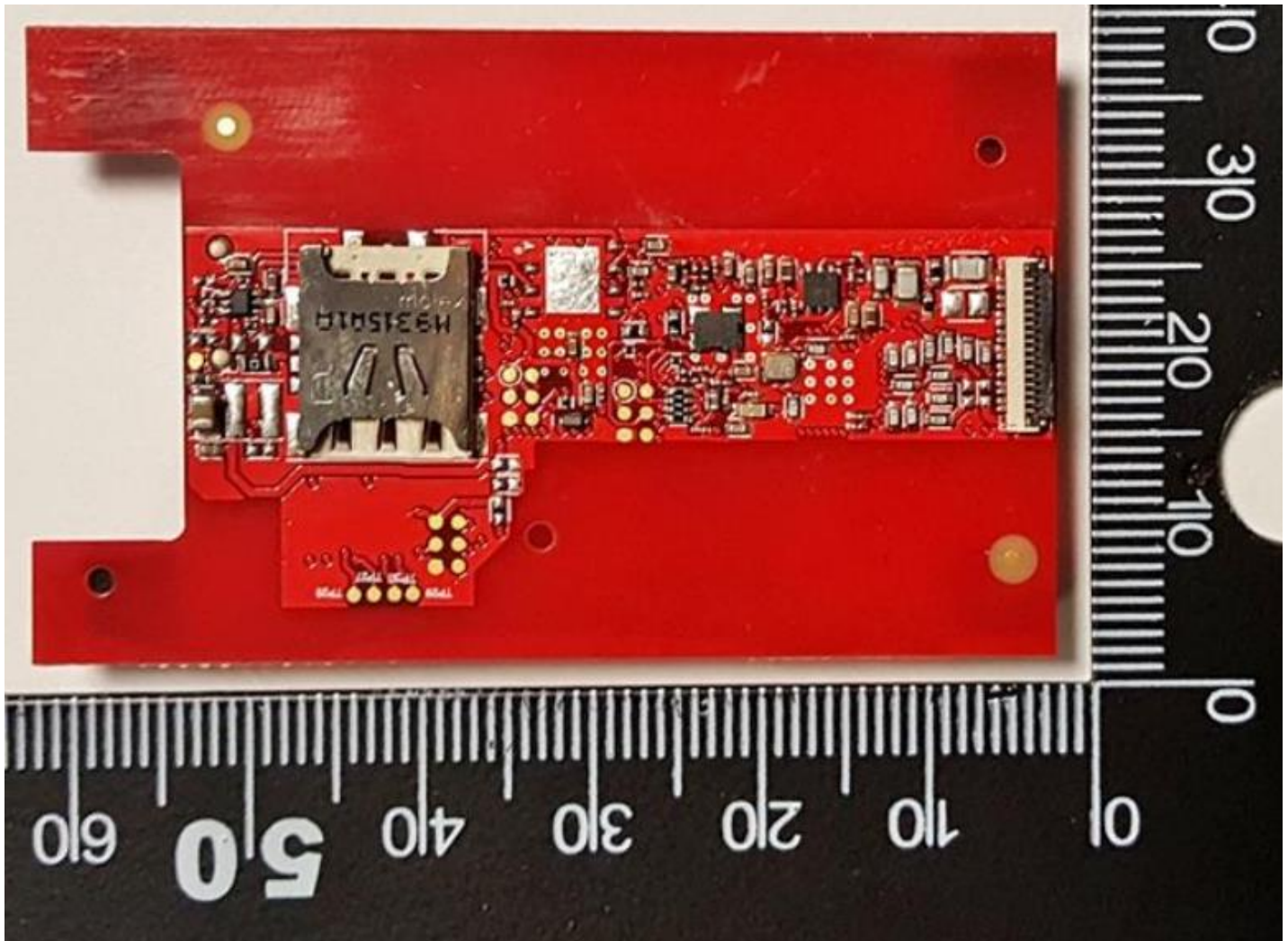
PCB-1080-03E Bottom Side
