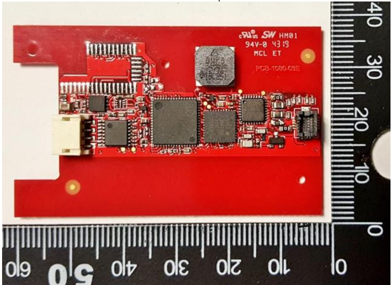
PCB-1080-03E Top Side
