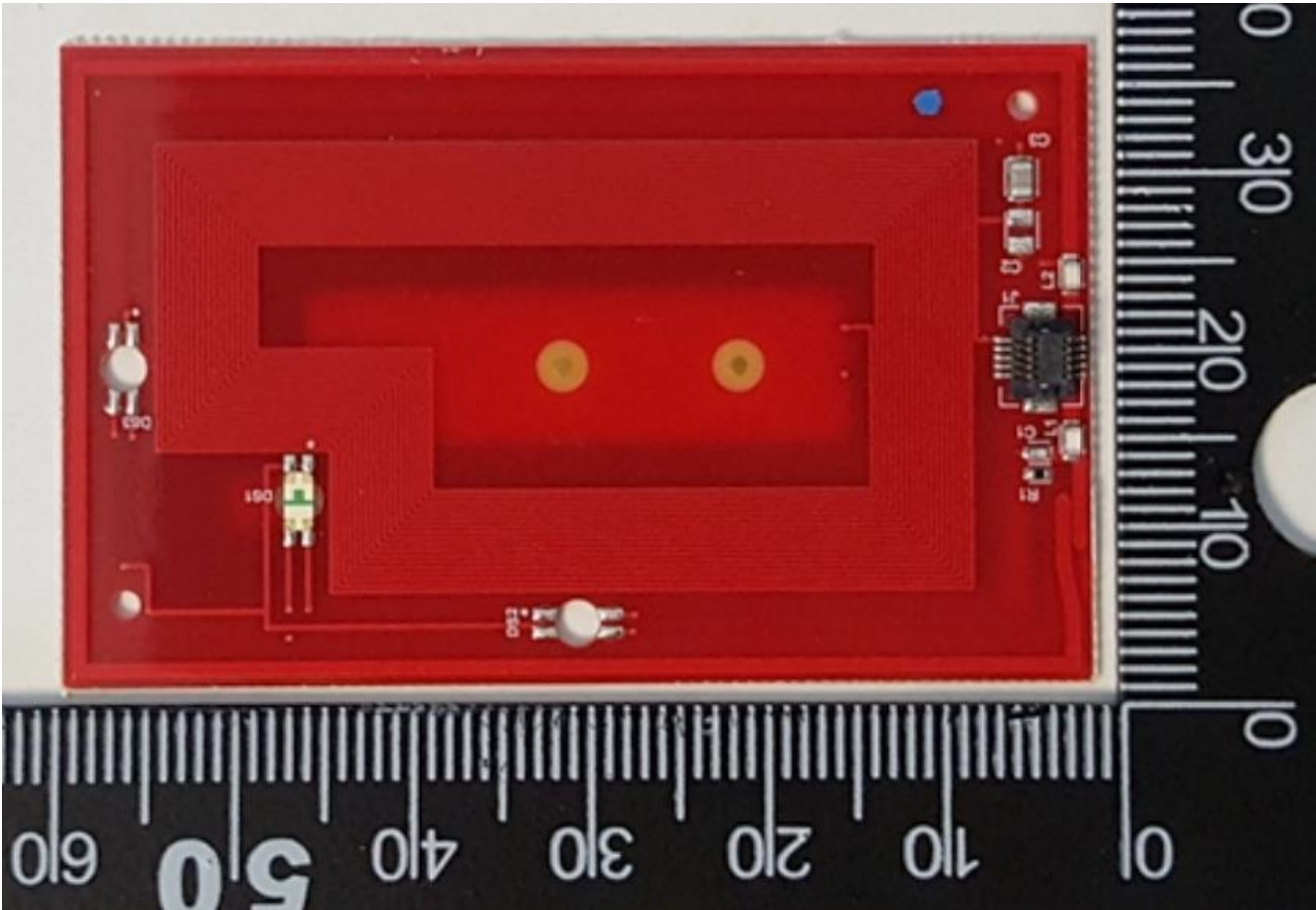
PCB-1098-05 Antenna
