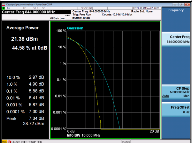
16QAM-20600
