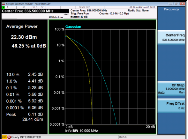
16QAM-20450
