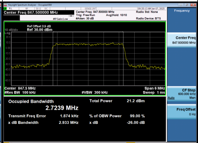
16QAM-27025
