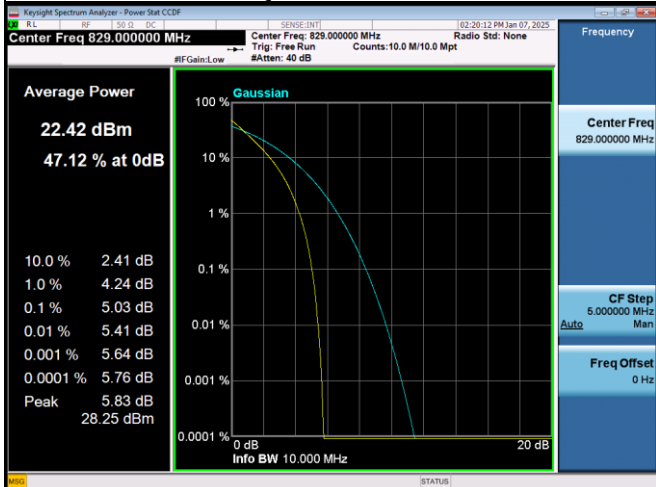
QPSK-20600
