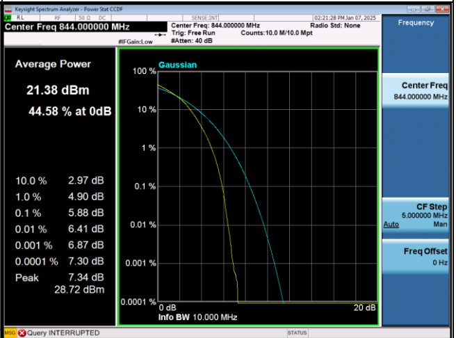
16QAM-20600
