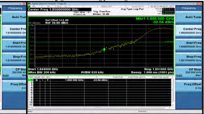
Band Edge_Band25 15MHz_QPSK 1 0_LowCH26115-1857.5
