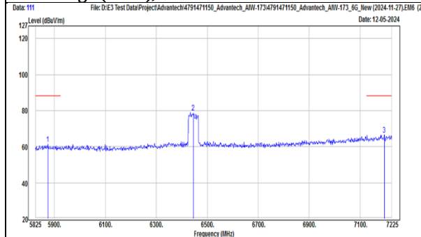
TX, 802.11be(EHT40) (Ch 99) Band Edge (Peak), Horizontal
