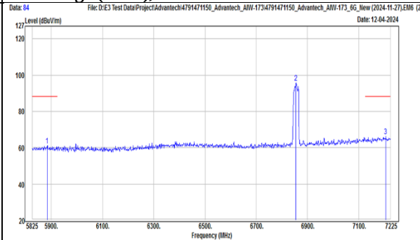
TX, 802.11be(EHT20) (Ch 181) Band Edge (Peak), Vertical
