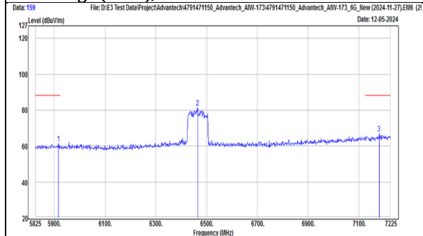
TX, 802.11be(EHT80) (Ch 103) Band Edge (Peak), Horizontal
