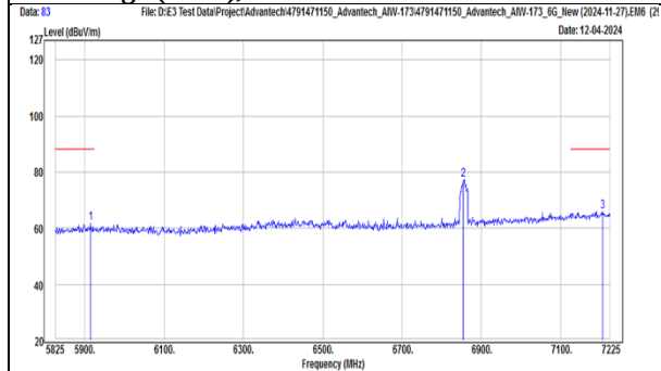
TX, 802.11be(EHT20) (Ch 181) Band Edge (Peak), Horizontal
