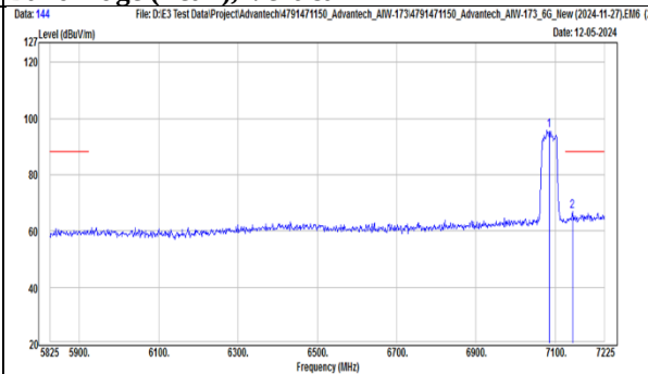
TX, 802.11be(EHT40) (Ch 227) Band Edge (Peak), Vertical
