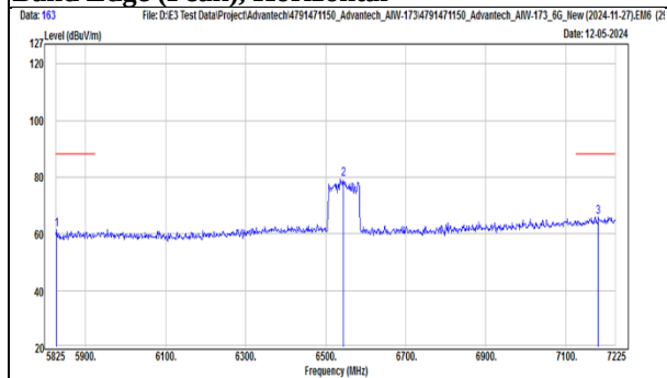
TX, 802.11be(EHT80) (Ch 119) Band Edge (Peak), Horizontal
