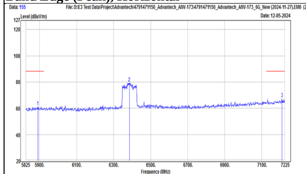
TX, 802.11be(EHT80) (Ch 87) Band Edge (Peak), Horizontal
