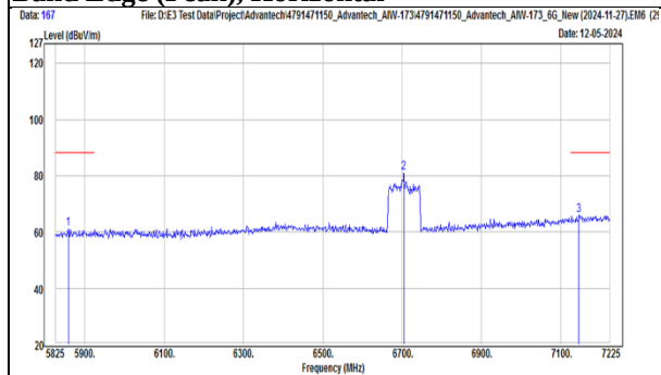
TX, 802.11be(EHT80) (Ch 151) Band Edge (Peak), Horizontal
