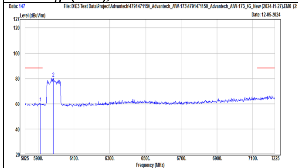
TX, 802.11be(EHT80) (Ch 7) Band Edge (Peak), Horizontal
