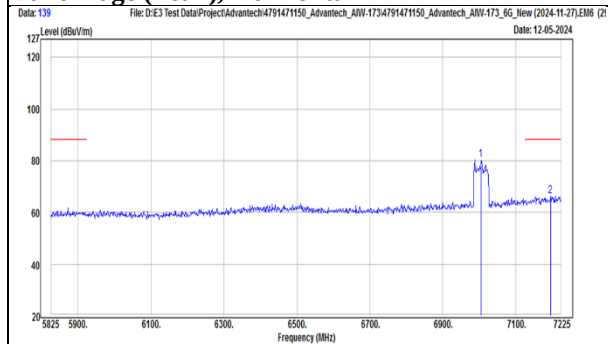
TX, 802.11be(EHT40) (Ch 211) Band Edge (Peak), Horizontal
