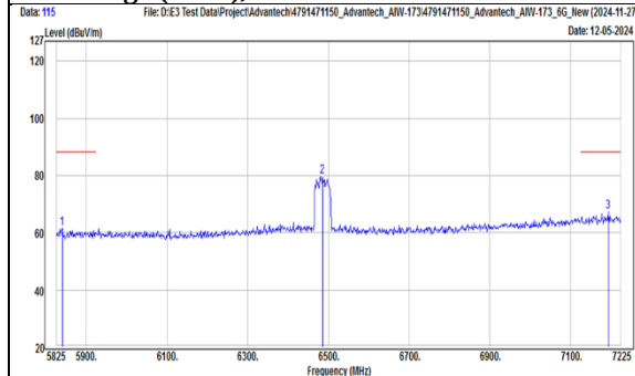
TX, 802.11be(EHT40) (Ch 107) Band Edge (Peak), Horizontal
