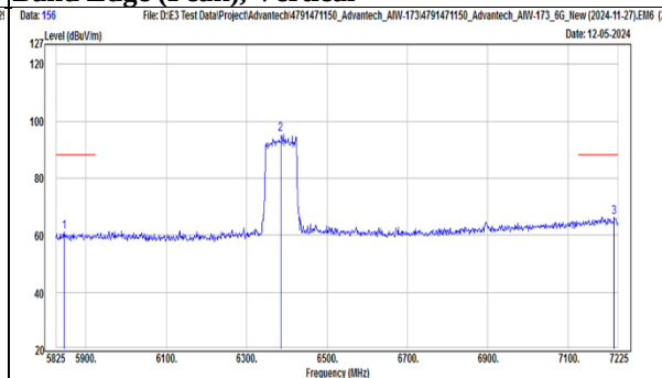
TX, 802.11be(EHT80) (Ch 87) Band Edge (Peak), Vertical
