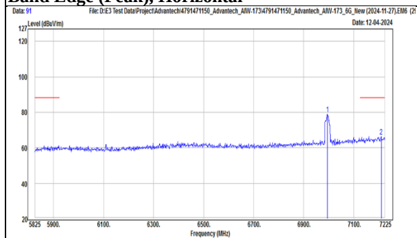
TX, 802.11be(EHT20) (Ch 209) Band Edge (Peak), Horizontal
