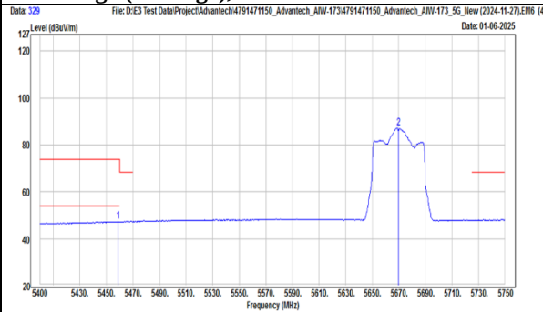
TX, 802.11be(EHT40) (Ch 134) Band Edge (Peak), Horizontal
