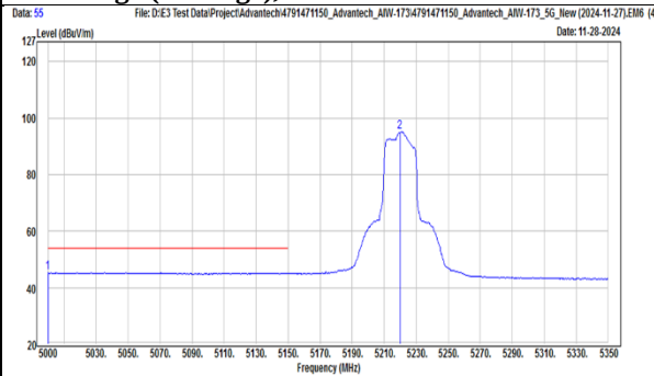
TX, 802.11be(EHT20) (Ch 44) Band Edge (Peak), Horizontal
