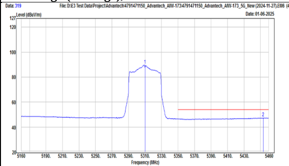
TX, 802.11be(EHT40) (Ch 62) Band Edge (Peak), Horizontal
