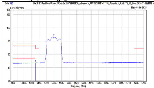
TX, 802.11be(EHT40) (Ch 102) Band Edge (Peak), Horizontal
