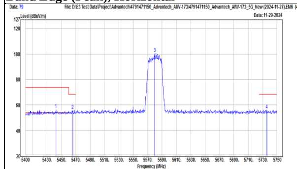
TX, 802.11be(EHT20) (Ch 116) Band Edge (Peak), Horizontal
