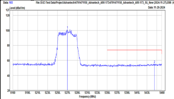
TX, 802.11be(EHT40) (Ch 54) Band Edge (Peak), Horizontal
