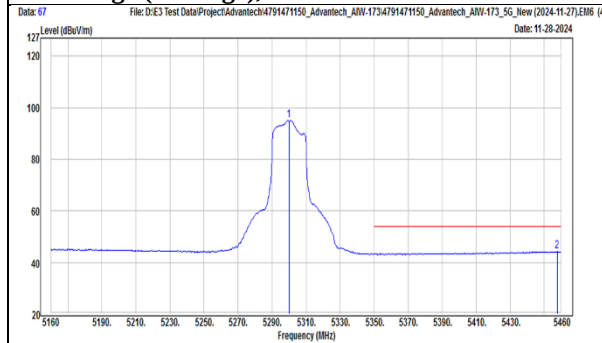
TX, 802.11be(EHT20) (Ch 60) Band Edge (Peak), Horizontal
