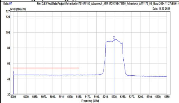
TX, 802.11be(EHT40) (Ch 46) Band Edge (Peak), Horizontal
