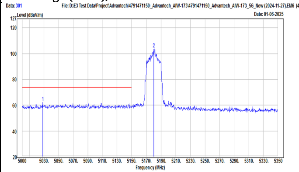
TX, 802.11be(EHT20) (Ch 36) Band Edge (Peak), Horizontal
