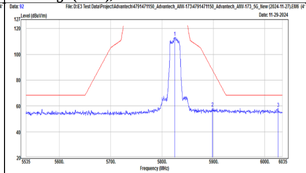
TX, 802.11be(EHT20) (Ch 165) Band Edge (Peak), Vertical
