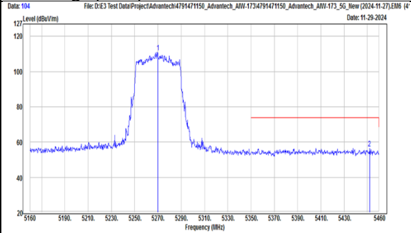
TX, 802.11be(EHT40) (Ch 54) Band Edge (Peak), Vertical
