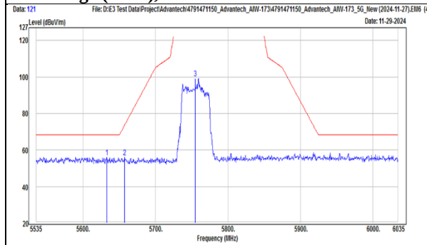
TX, 802.11be(EHT40) (Ch 151) Band Edge (Peak), Horizontal
