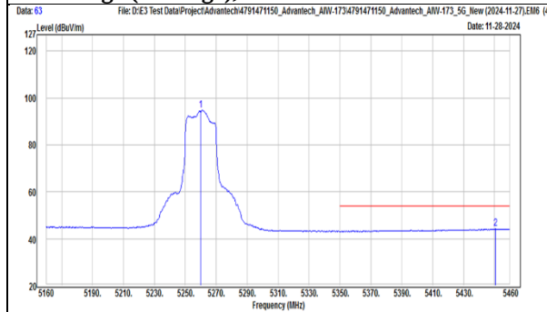
TX, 802.11be(EHT20) (Ch 52) Band Edge (Peak), Horizontal
