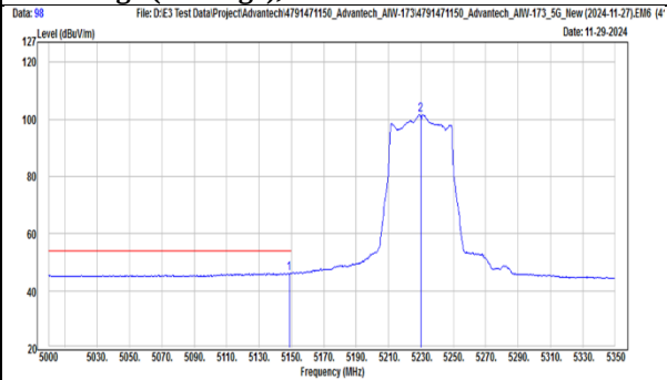
TX, 802.11be(EHT40) (Ch 46) Band Edge (Peak), Vertical
