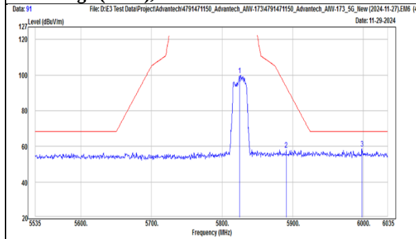
TX, 802.11be(EHT20) (Ch 165) Band Edge (Peak), Horizontal
