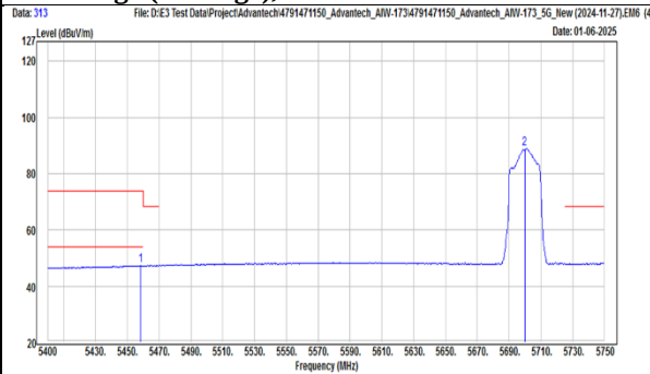
TX, 802.11be(EHT20) (Ch 140) Band Edge (Peak), Horizontal
