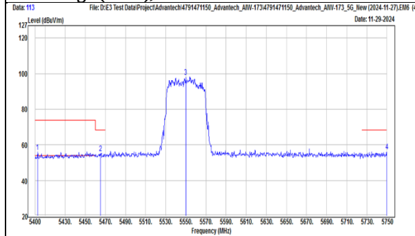
TX, 802.11be(EHT40) (Ch 110) Band Edge (Peak), Horizontal
