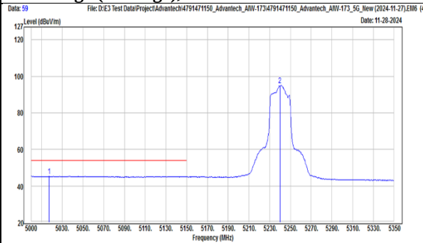
TX, 802.11be(EHT20) (Ch 48) Band Edge (Peak), Horizontal
