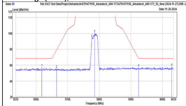
TX, 802.11be(EHT20) (Ch 157) Band Edge (Peak), Horizontal
