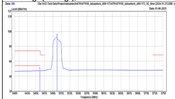
TX, 802.11be(EHT20) (Ch 100) Band Edge (Peak), Horizontal
