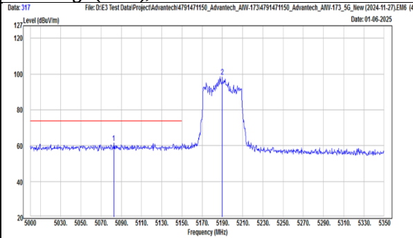
TX, 802.11be(EHT40) (Ch 38) Band Edge (Peak), Horizontal
