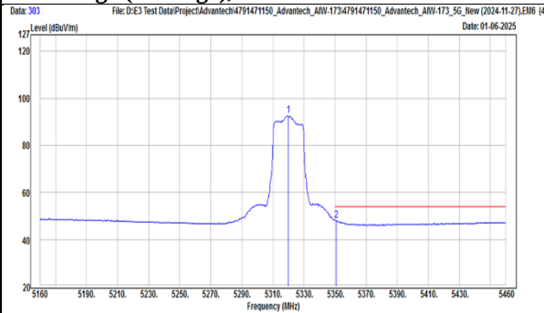
TX, 802.11be(EHT20) (Ch 64) Band Edge (Peak), Horizontal
