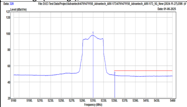
TX, 802.11be(EHT40) (Ch 62) Band Edge (Peak), Vertical
