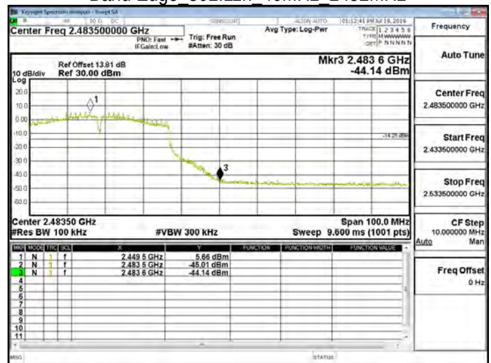
Band Edge 802.11n 40MHz 2452MHz
