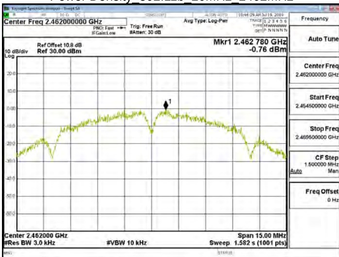
Power Density 802.11b 20MHz 2462MHz
