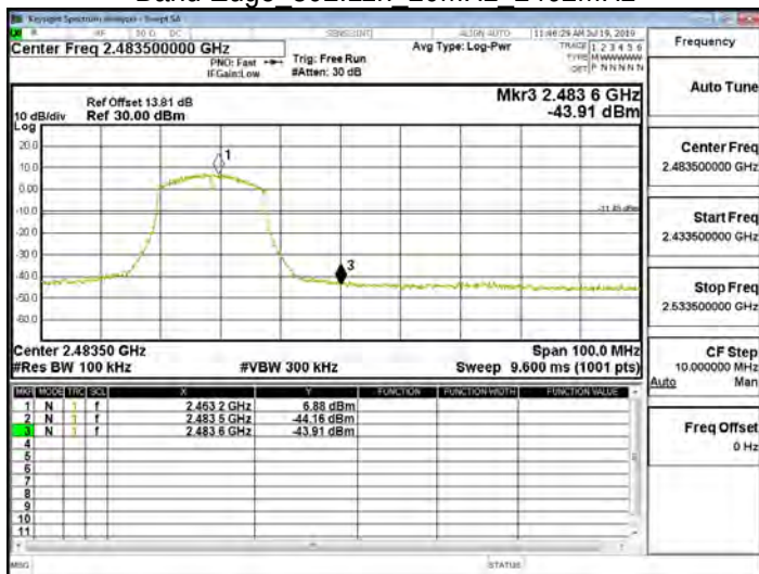
Band Edge 802.11n 20MHz 2462MHz
