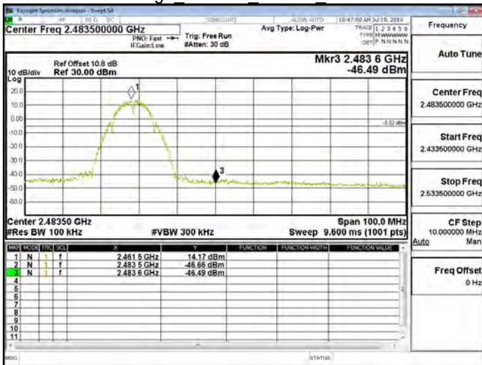
Band Edge 802.11b 20MHz 2462MHz
