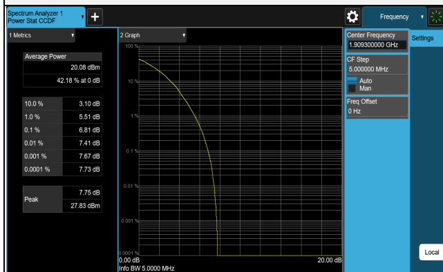
64QAM CH 19193 (1909.3MHz)
