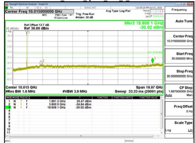
Band2 20MHz QPSK RB1 0 CH19100
