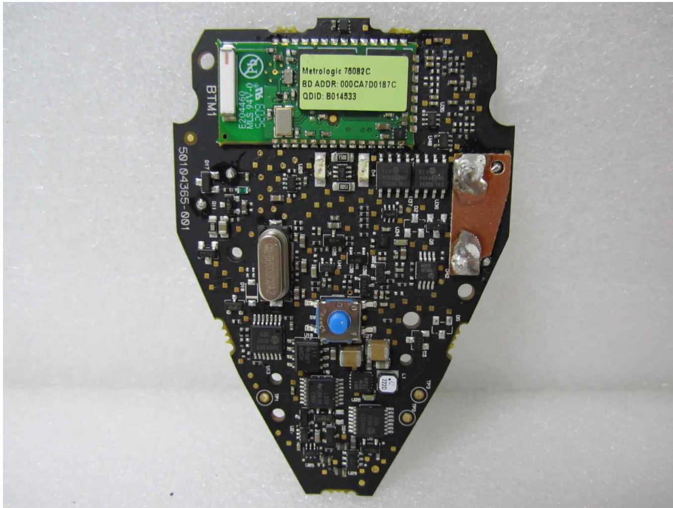
메인보드 전면
