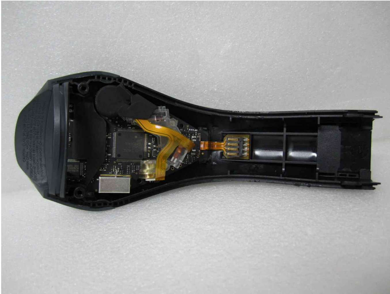
내부
