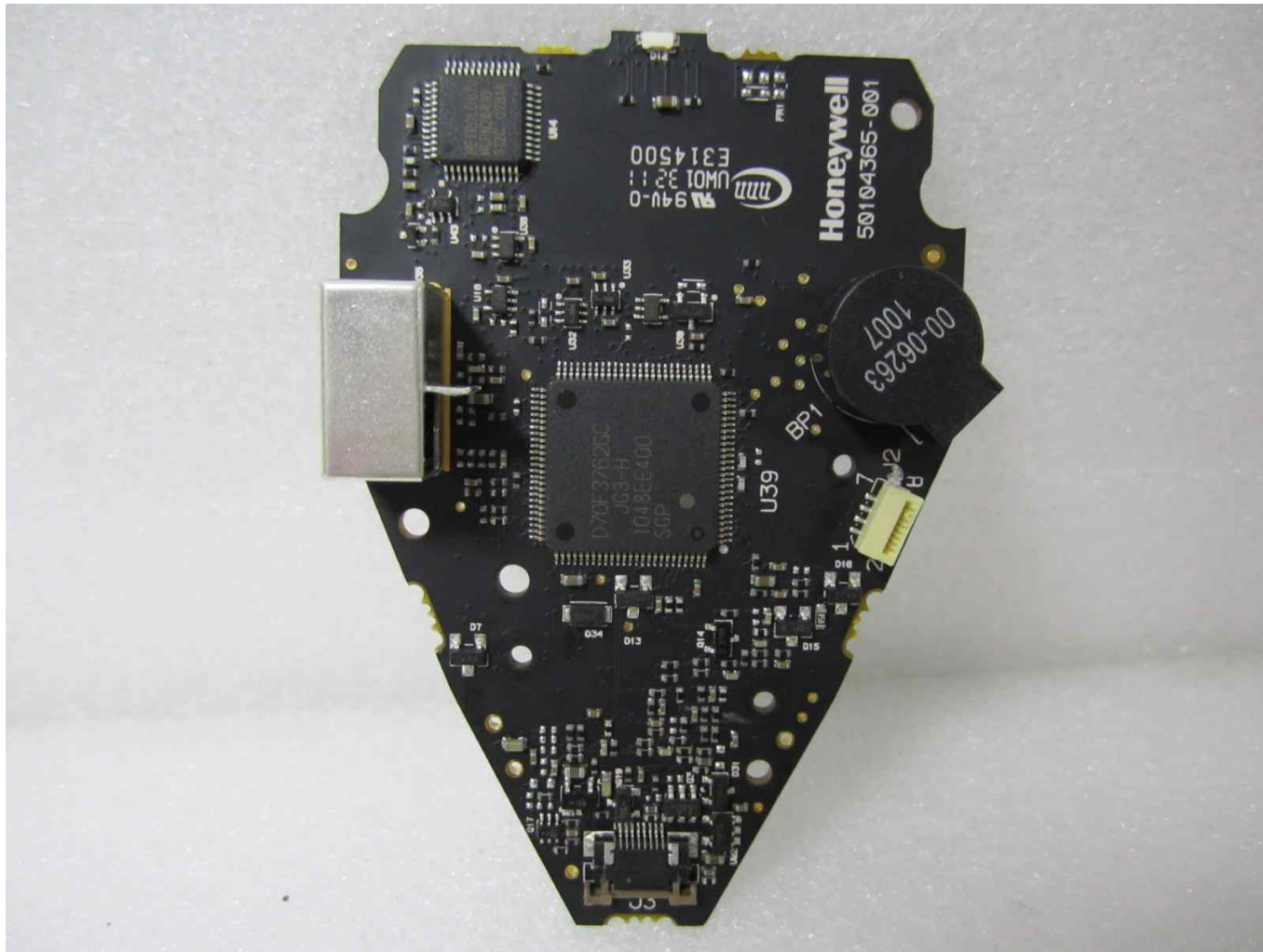
메인보드 후면
