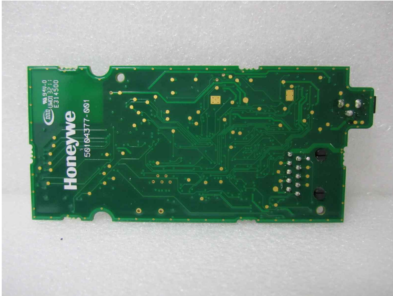
메인보드 후면
