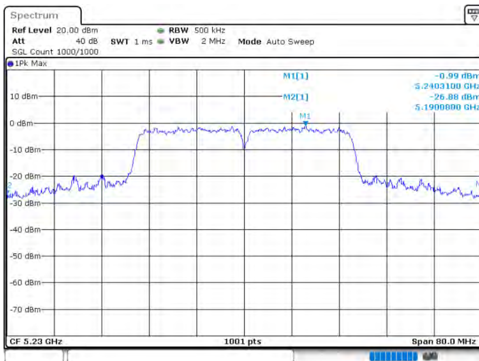
-26 dB BW NVNT 802.11n(HT40) 5230MHz Ant 3
