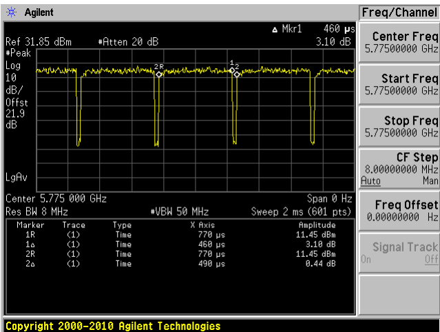
802.11VHT80 mode
