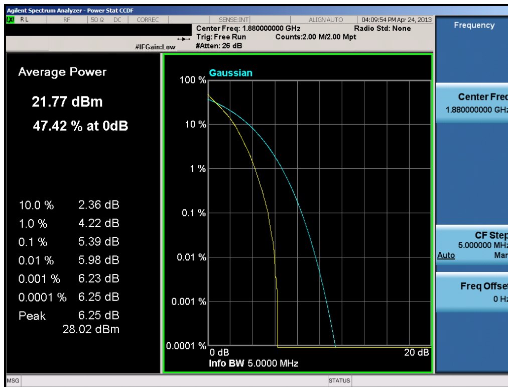
Plot 10-7. PAR Plot (5.0MHz QPSK – RB Size 25)
