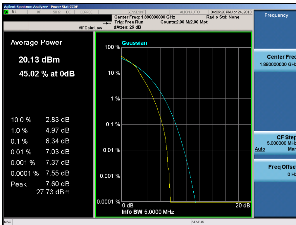
Plot 10-8. PAR Plot (5.0MHz 16-QAM – RB Size 25)
