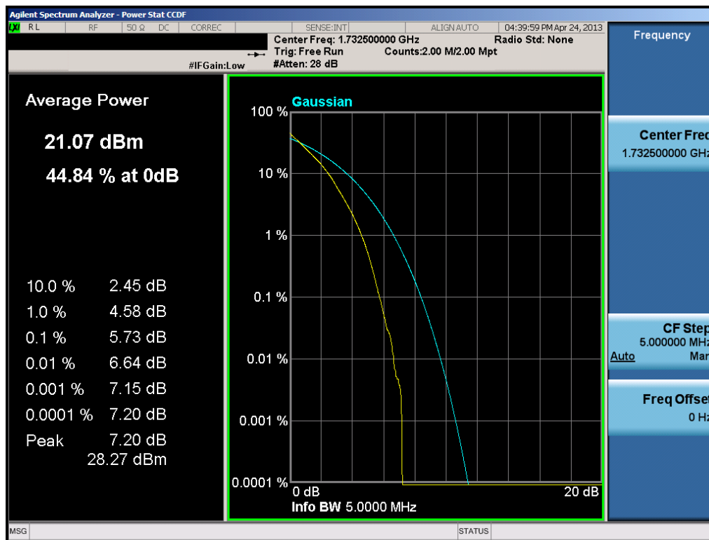
Plot 9-7. PAR Plot (5.0MHz QPSK – RB Size 25)
