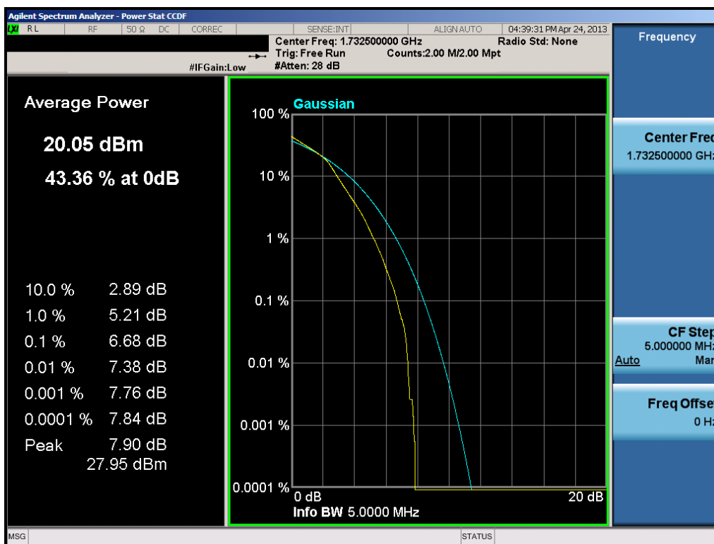
Plot 9-8. PAR Plot (5.0MHz 16-QAM – RB Size 25)
