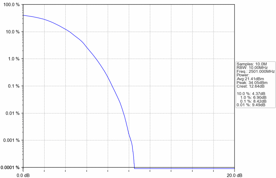
Band41 10MHz 64QAM LCH 2501MHz RB 50 0 NTNV
