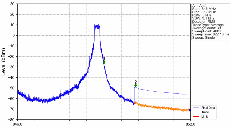
Band26b_3MHz_QPSK_HCH_847.5MHz_RB_1_14_NTNV
