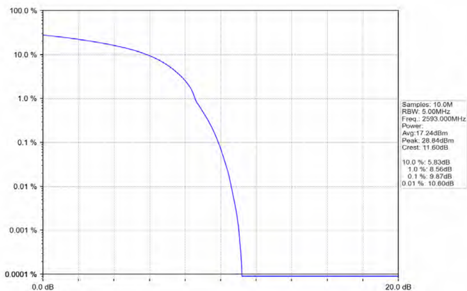
Band41_20MHz_QPSK_MCH_2593MHz_RB_100_0_NTNV
