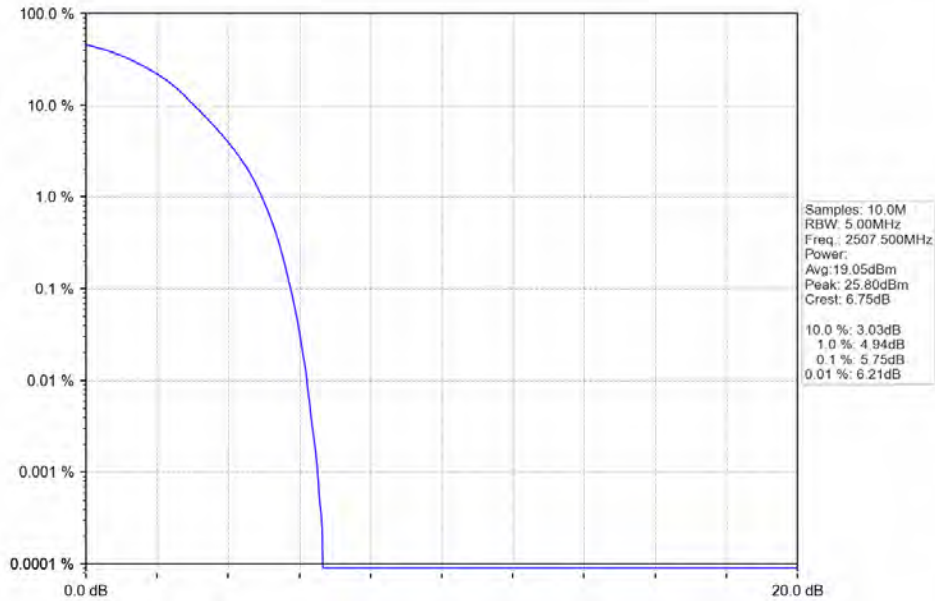
Band7 15MHz QPSK LCH 2507.5MHz RB 75 0 NTNV
