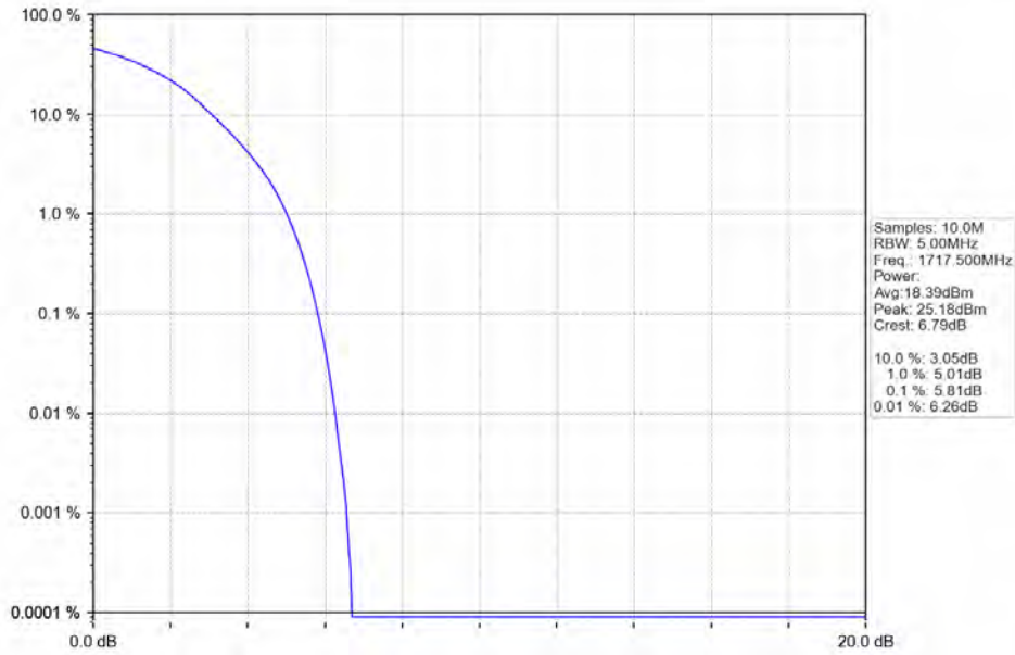
Band 4 15MHz QPSK LCH 1717.5MHz RB 75 0 NTN
