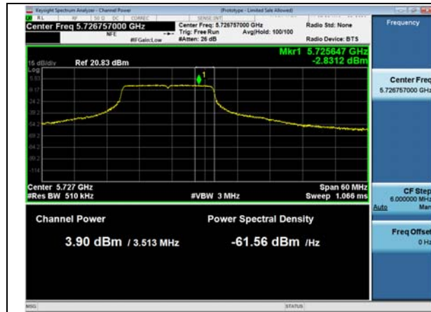
Antenna A
