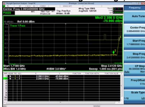
Antenna A
