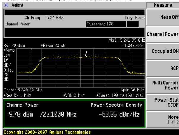
Antenna A
