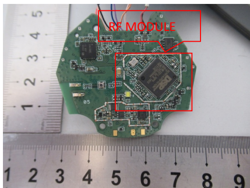
CP-HS-WL-562-N-US -PCB 2
