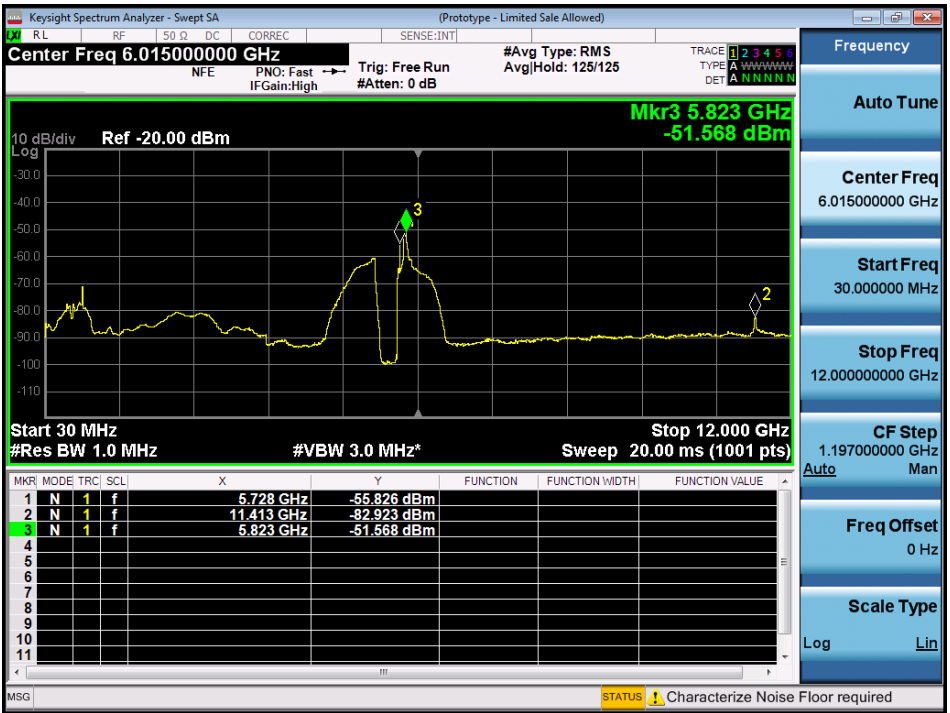
Antenna A
