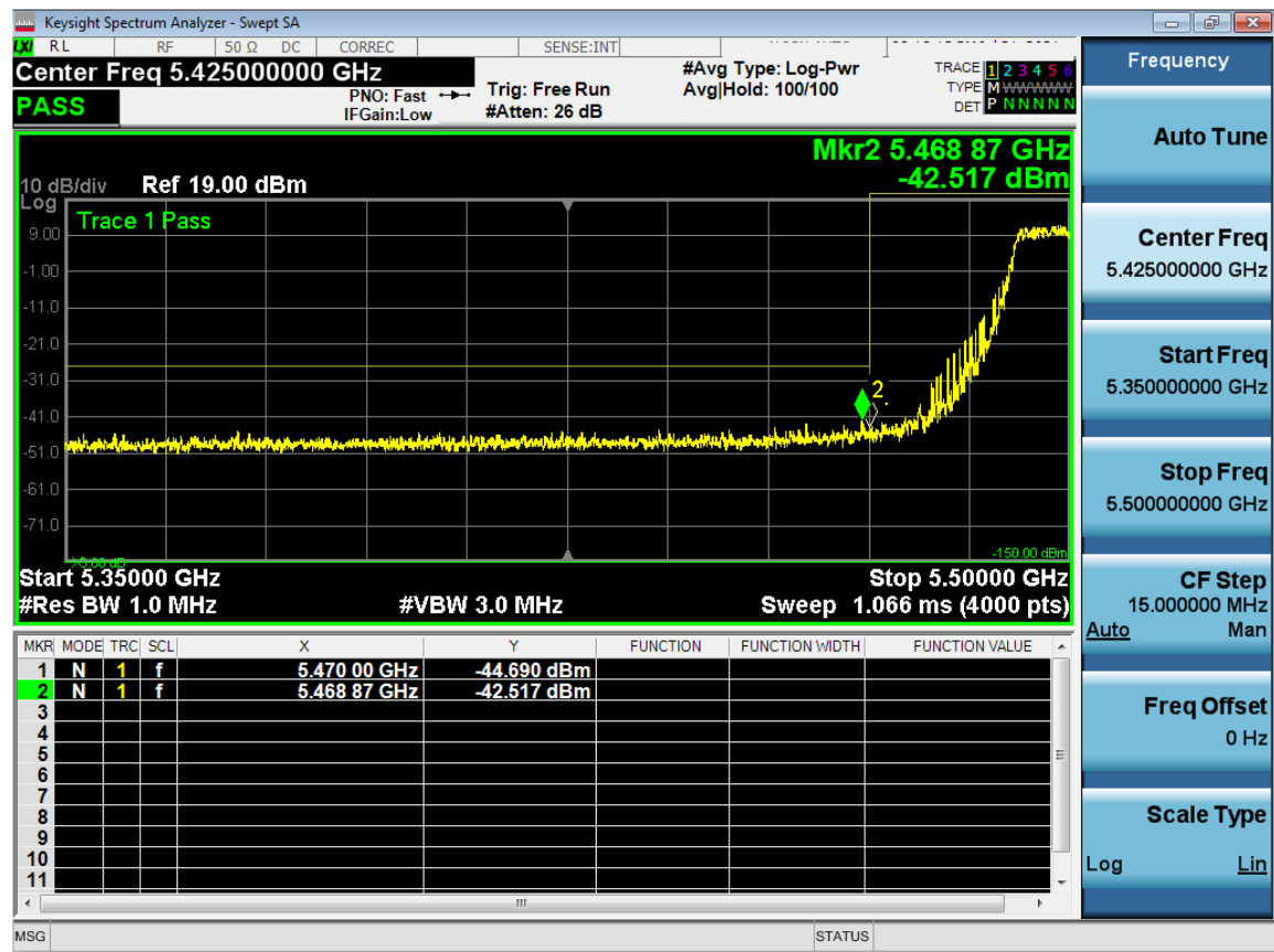
Antenna A
