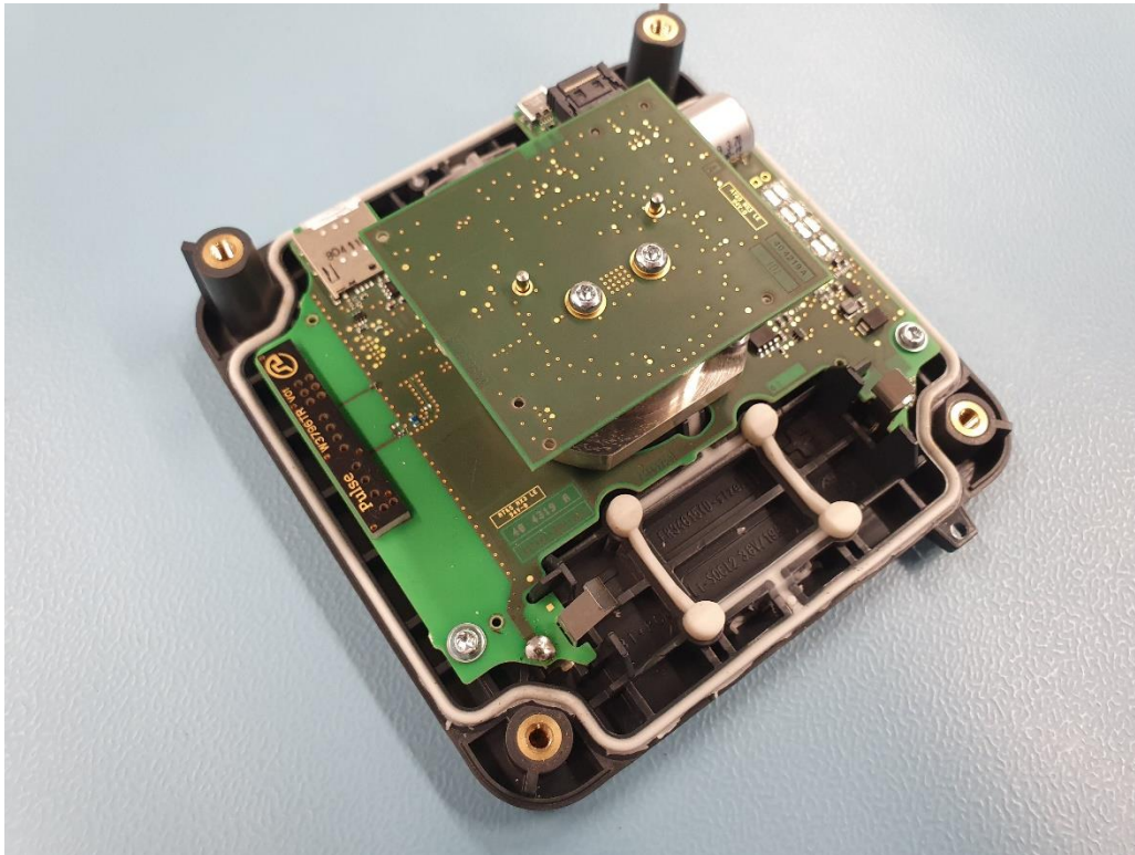
Subassembly FWR30:
