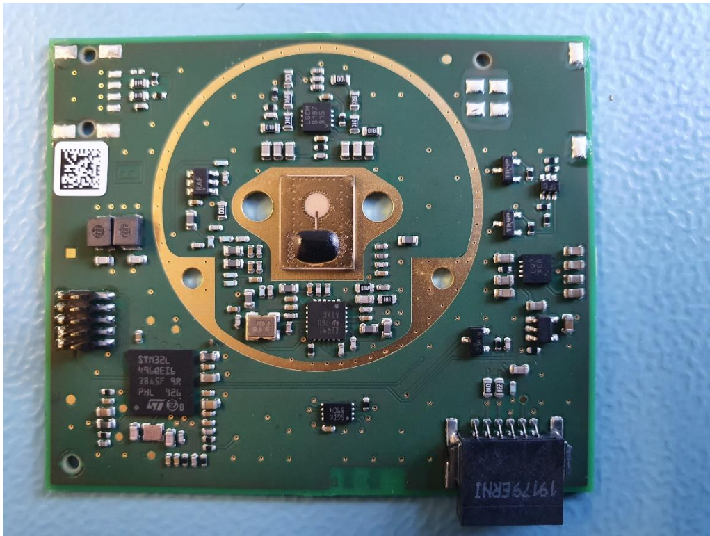
Sensor module top:
