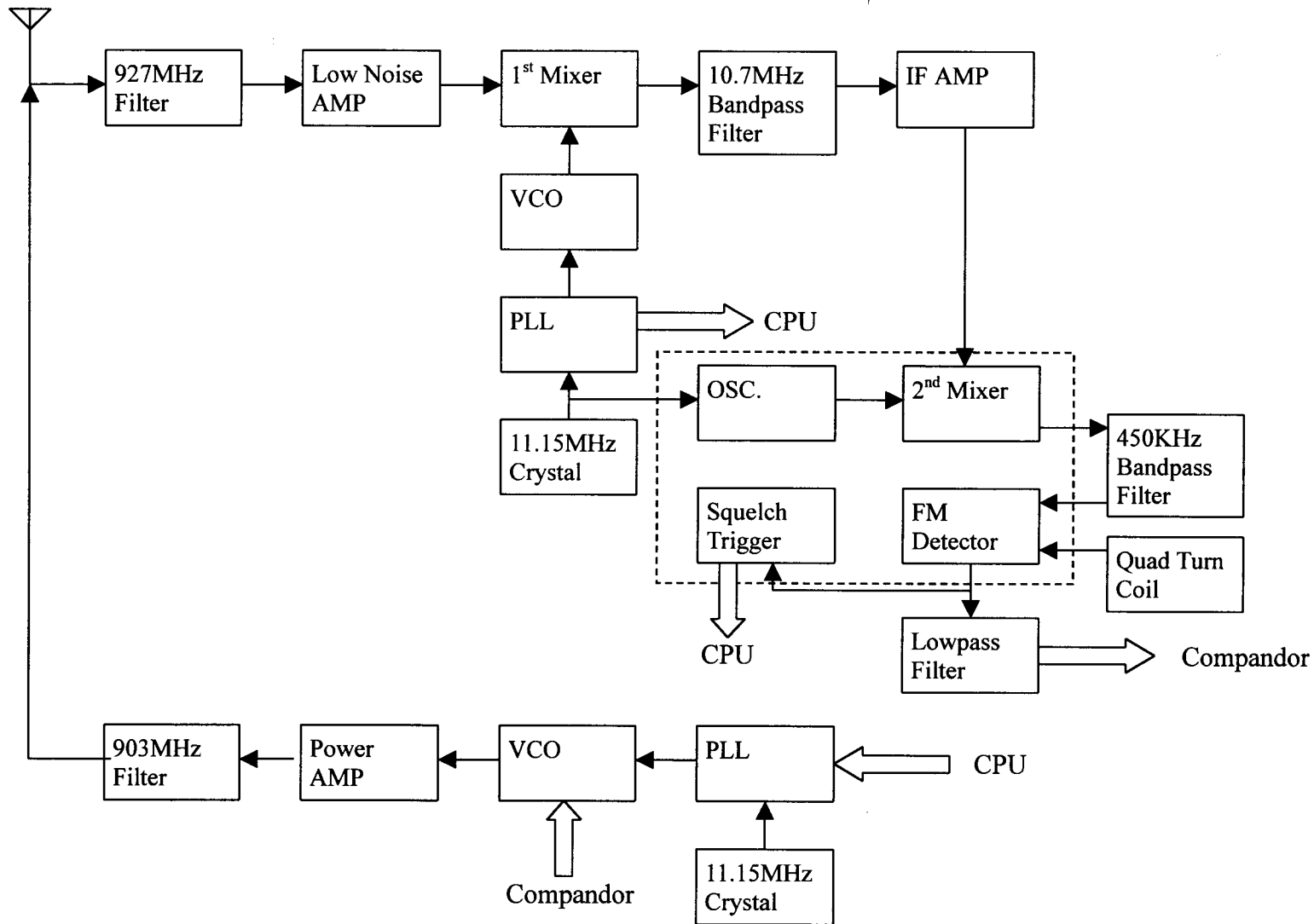
FF2125/FF2150 900MHz phone base RF module block diagram
