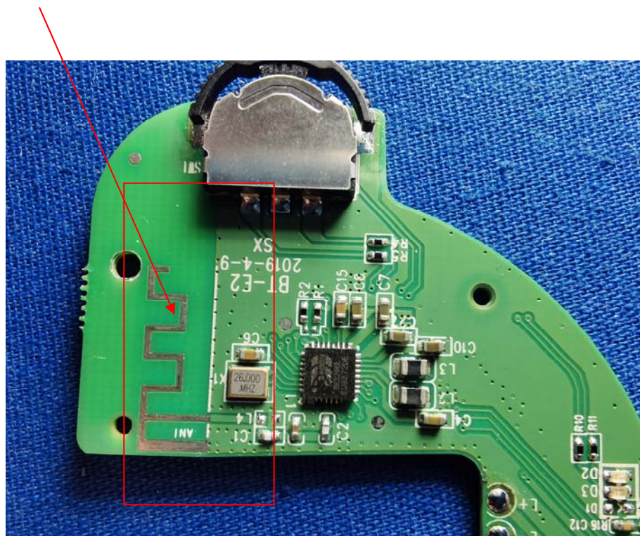
Antenna
