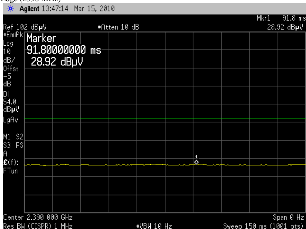
Plot 2 : Band Edge (2390 MHz)
