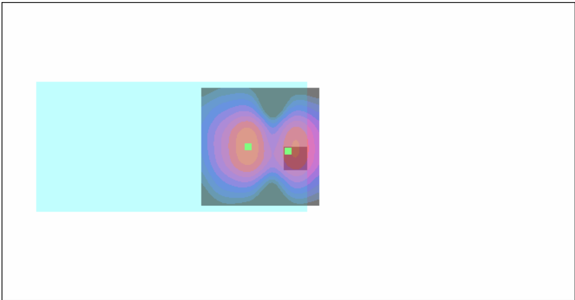
Radial L; CDMA1900; 1.025 KHz sinusoidal
