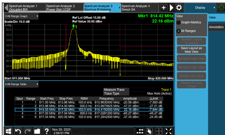
1RB#0 CH 26705 (815.5 MHz)
