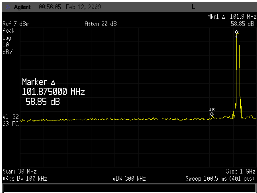
Out-of-band: 30-1000MHz
