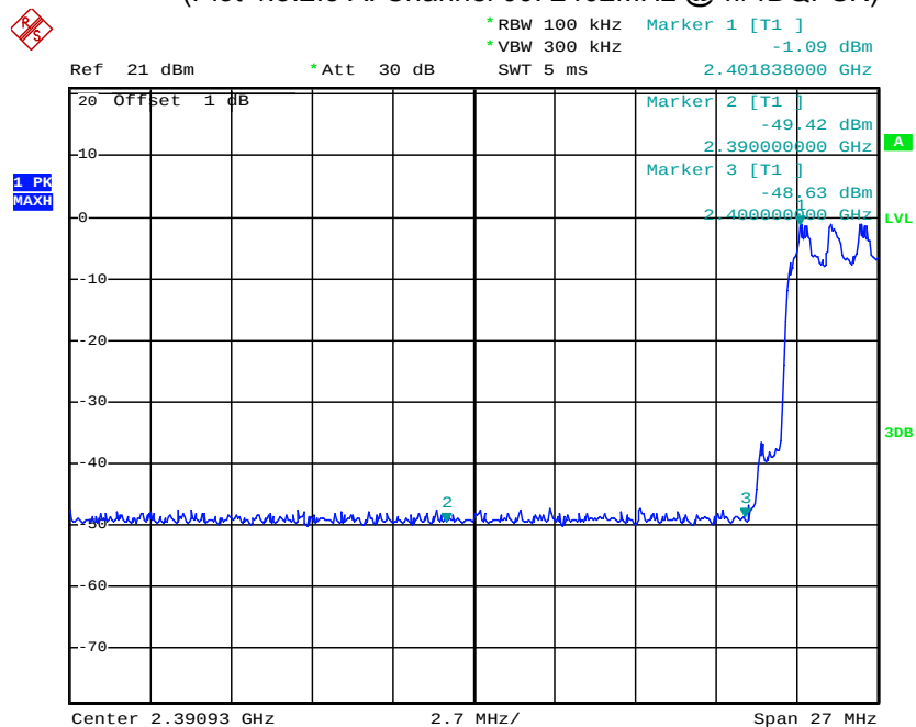
(Plot 4.5.2.3 A: Channel 00: 2402MHz @ \pi/4 DQPSK)
