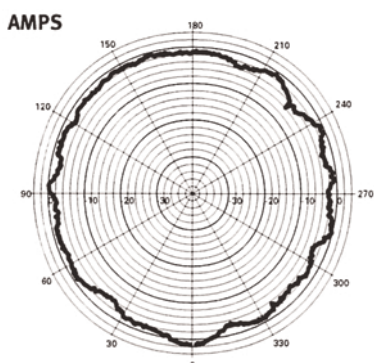
Typisches Strahlungsdiagramm (H-Ebene) Typical radiation pattern (H-plane)
