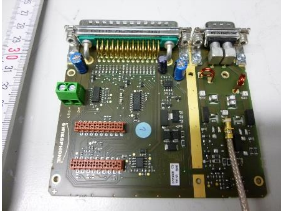
Photo 47: RF module
