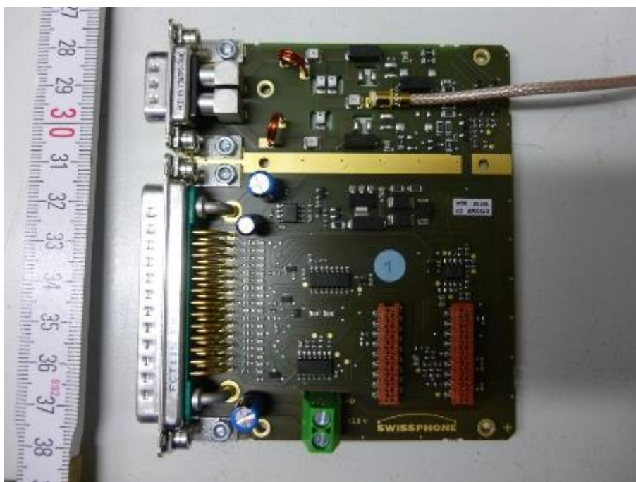
Photo 46: RF module
