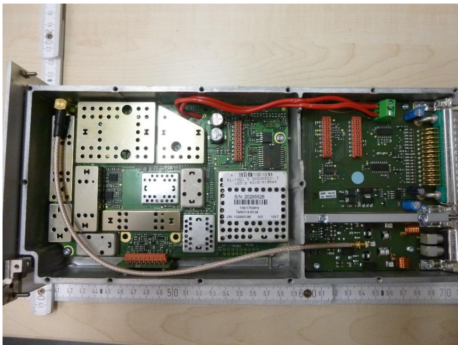
Photo 42: RF module
