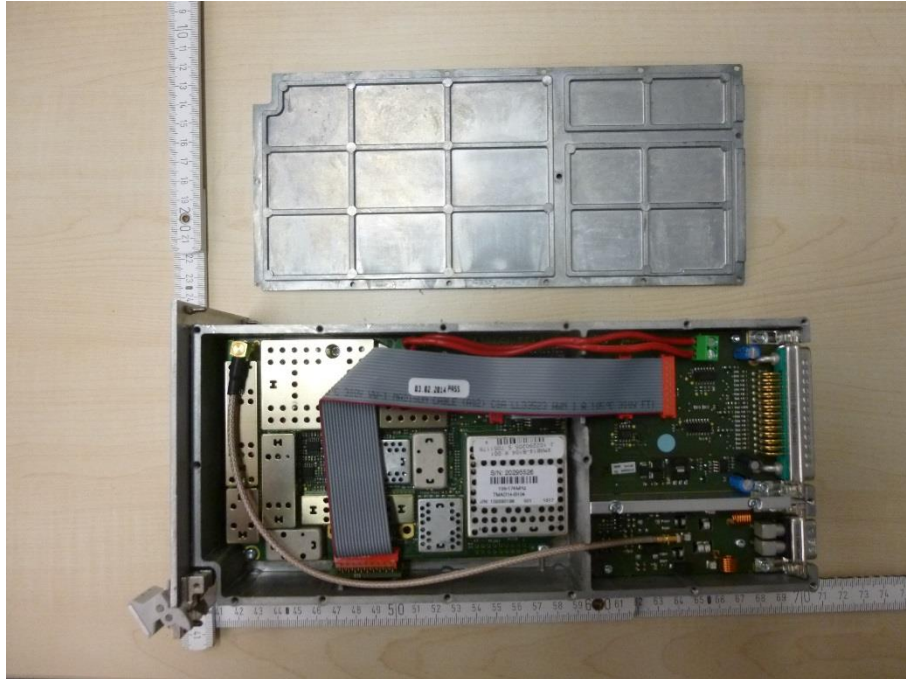
Photo 39: RF module
