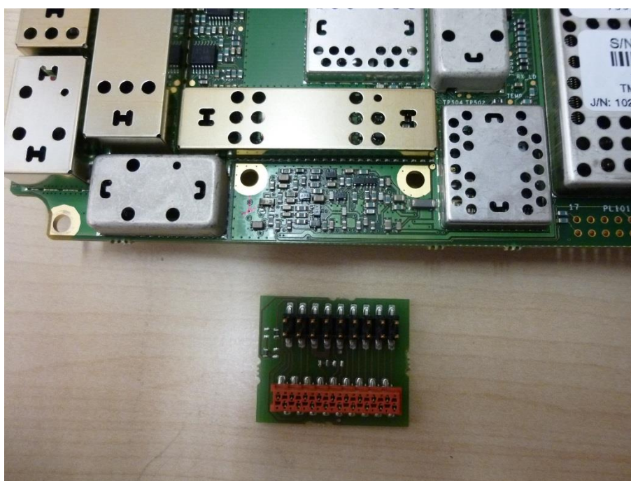
Photo 46: RF module
