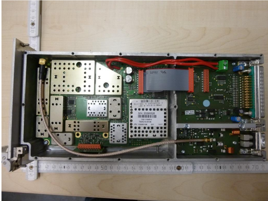
Photo 41: RF module
