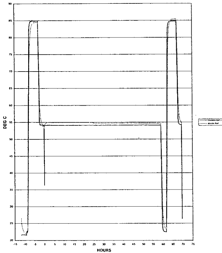
SN2007 HOT LIFE TEST
