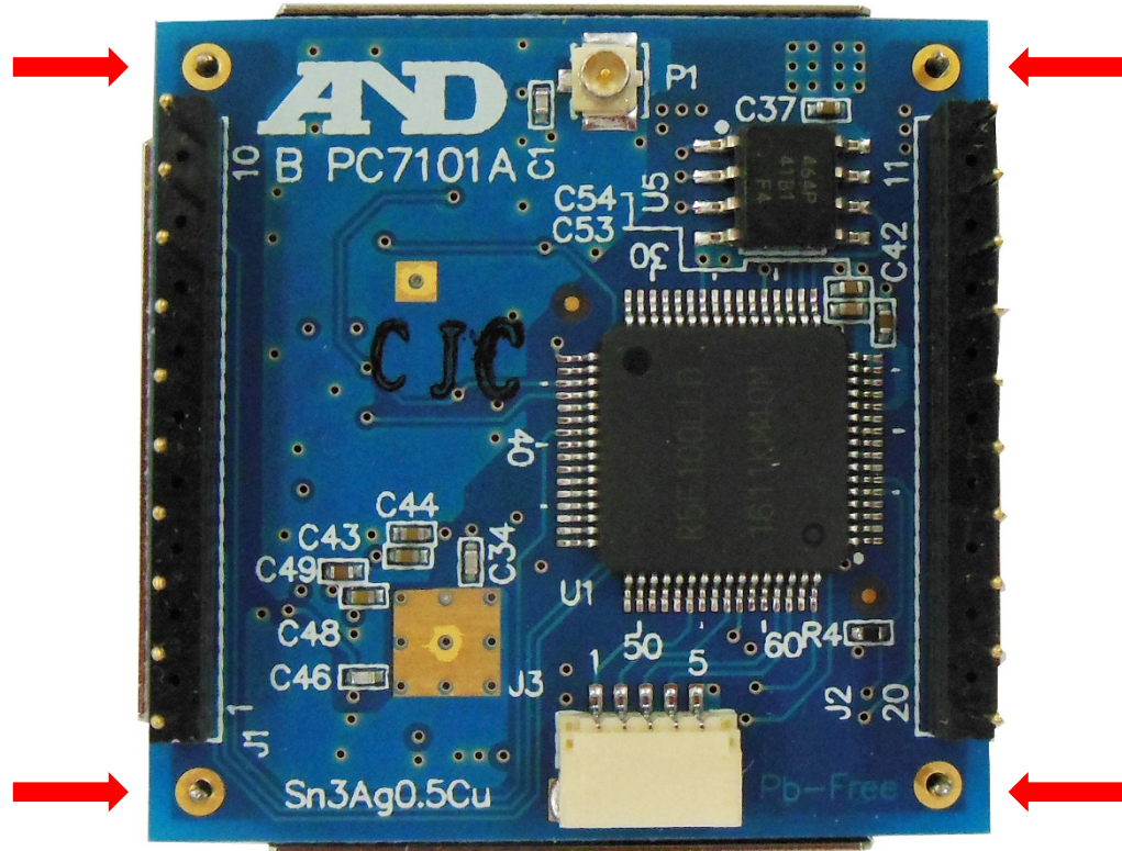
裏側シールドケース付き Bottom w/shield case
