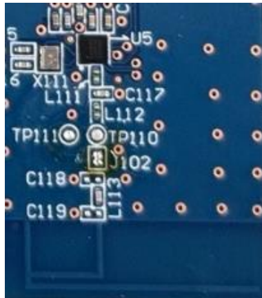
Bluetooth IC & PCB Antenna
