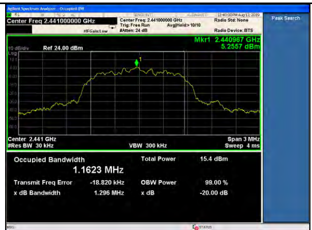
BT- \pi/4 DQPSK-20 dB BW-Mid
