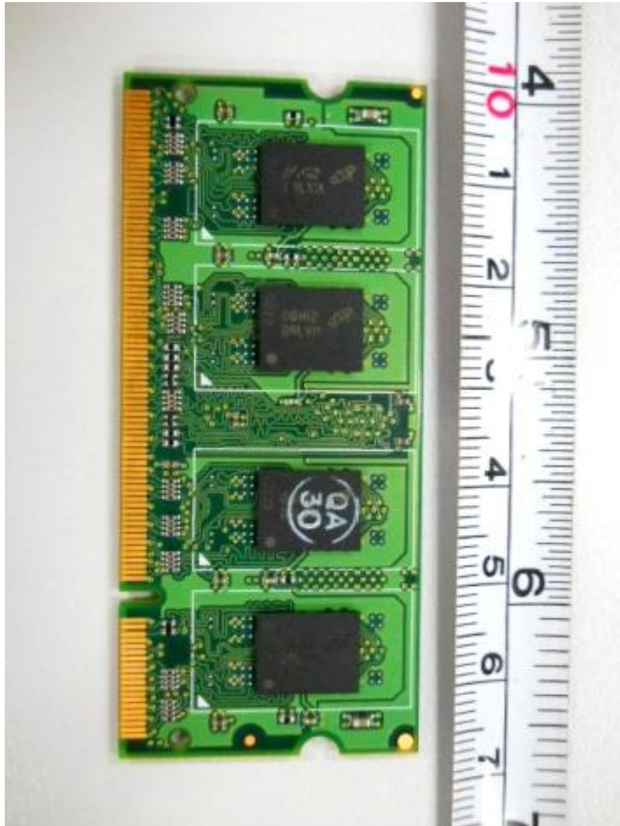
DDR2-SODIMM PCB Trace Side
