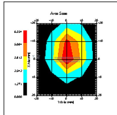
5600MHz
