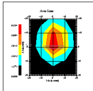
5800MHz
